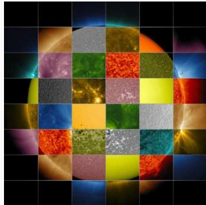
Un collage di immagini del Sole a varie lunghezze d'onda realizzate da SDO. Crediti: NASA/SDO /Goddard Space Flight Center
